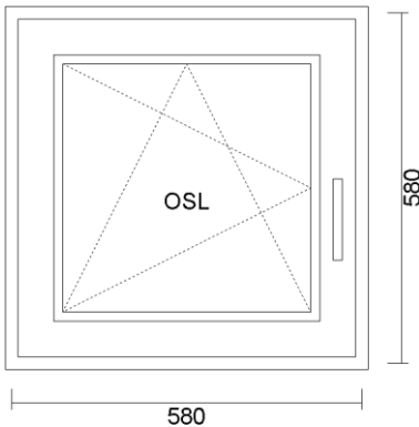
8) OKNO PVC (OSL). 580x580 Pohľad z vnútra
