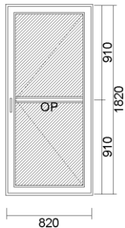
9) DVB PVC(OP)KĽUČKY,AL.PRAH.ZÁMO 820x1820 Pohľad z vnútra
